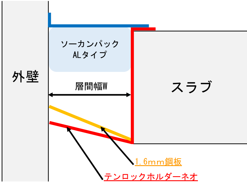
納まり図
